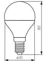
BILO 6,5W T SMD E14
