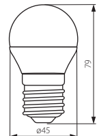
BILO 6,5W T SMD E27
