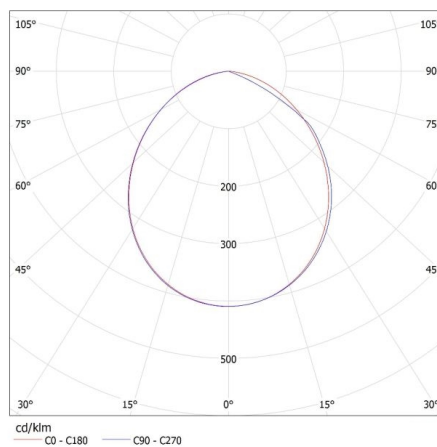
KANLUX S.A. (kat 23550) SEVIA LED 26 / Krzywa rozsytu światła (biegunowo)
