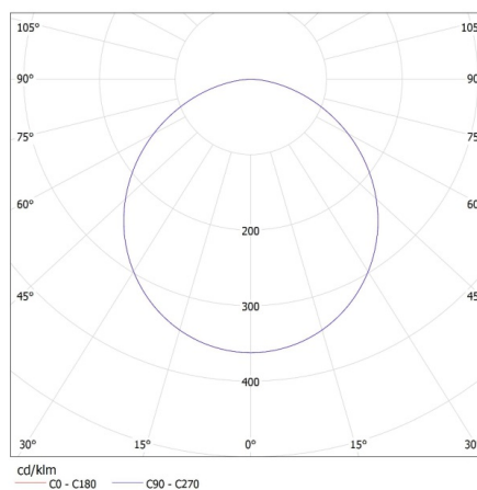
KANLUX S.A. (kat 25562) LITEN LED 8W-WW / Krzywa rozsyłu światła (biegunowo)
