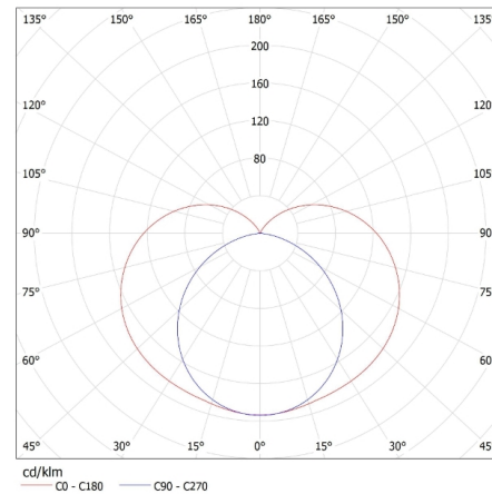
KANLUX S.A. (kat 27533) PESSA LED IP44 17W-NW / LDC (Polar)
