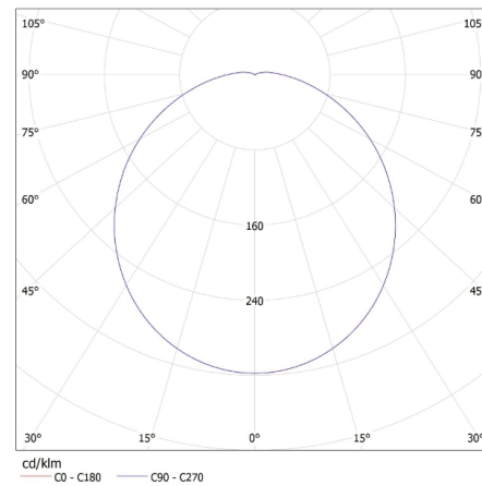
MILED0 (kat 31093) DUNO LED N24W-NW-O / LDC (Polar)
