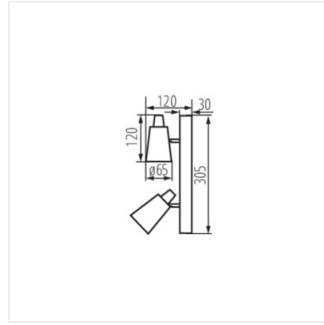
SEMPRA EL-2I
