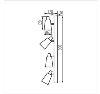
SEMPRA EL-4I
