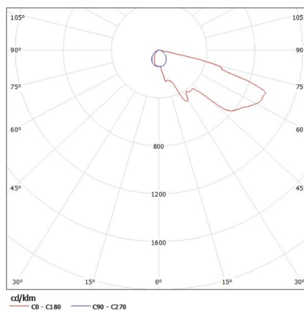
KANLUX S.A. (kat 4681) LINDA LED-J02 / Krzywa rozsyłu światła (biegunowo)
